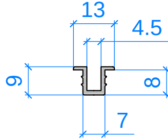
профиль space L=3000mm
