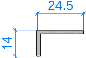
уголок 25x14 L=3000mm
