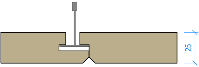
Кромка СК (скрытая). Применяется для монтажа с подвесной системой T24.
