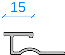
профиль step завершающий L=3000mm
