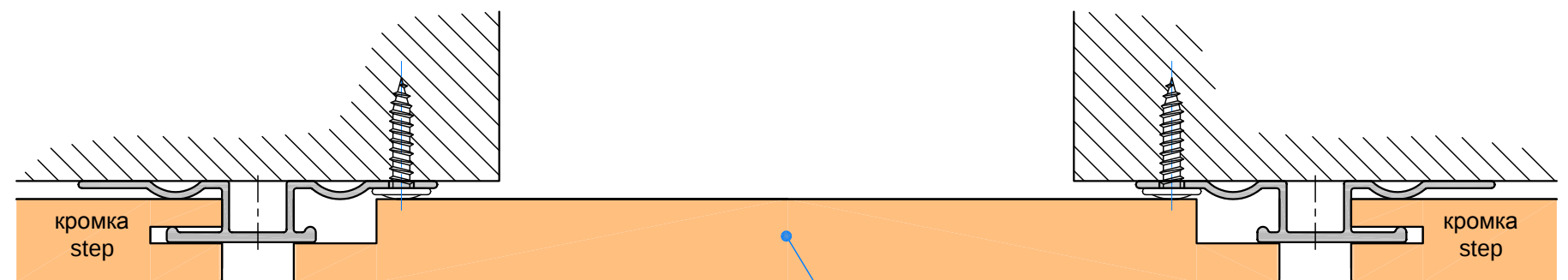
СЪЕМНАЯ ПАНЕЛЬ - ВИД СВЕРХУ
