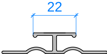
профиль seam разделительный L=3000mm
