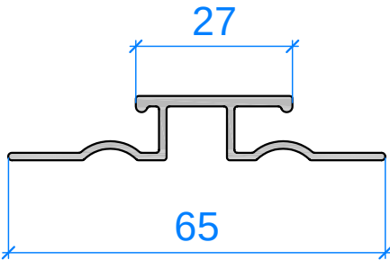
профиль step разделительный L=3000mm
