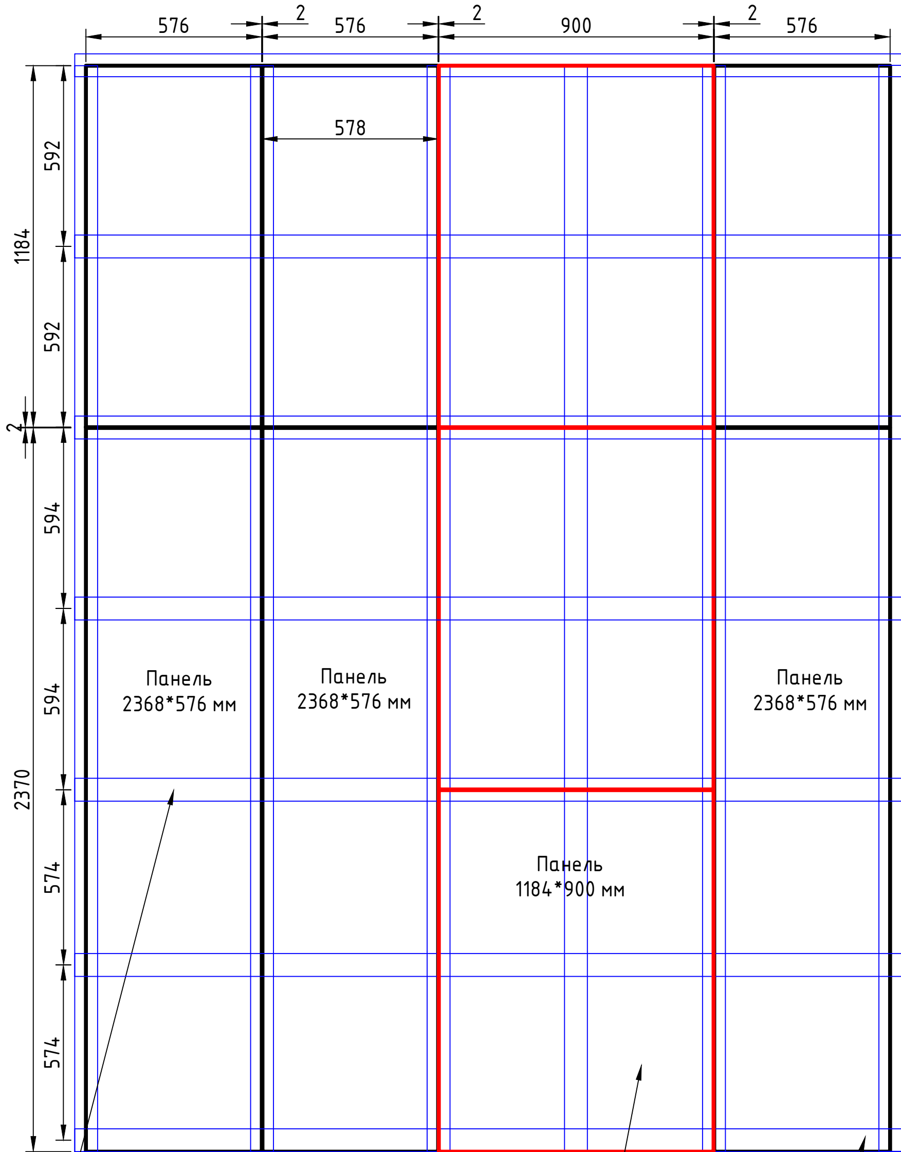
Пример сетки каркаса для акустических и декоративных панелей TAGinterio
